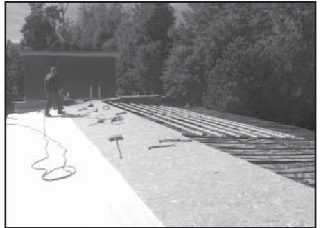
Montáž nových vrstev
